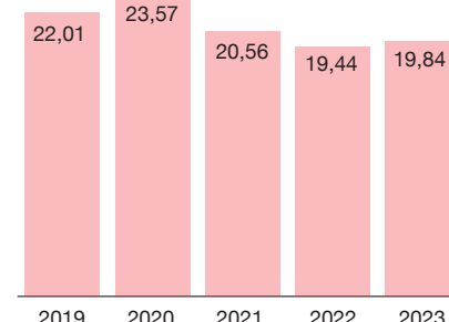
Wärmebedarf Produktion in kWh/hl prod. EG
