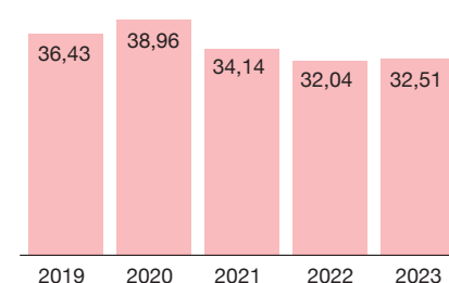
Gesamter Energieaufwand Produktion in kWh/hl prod. EG
